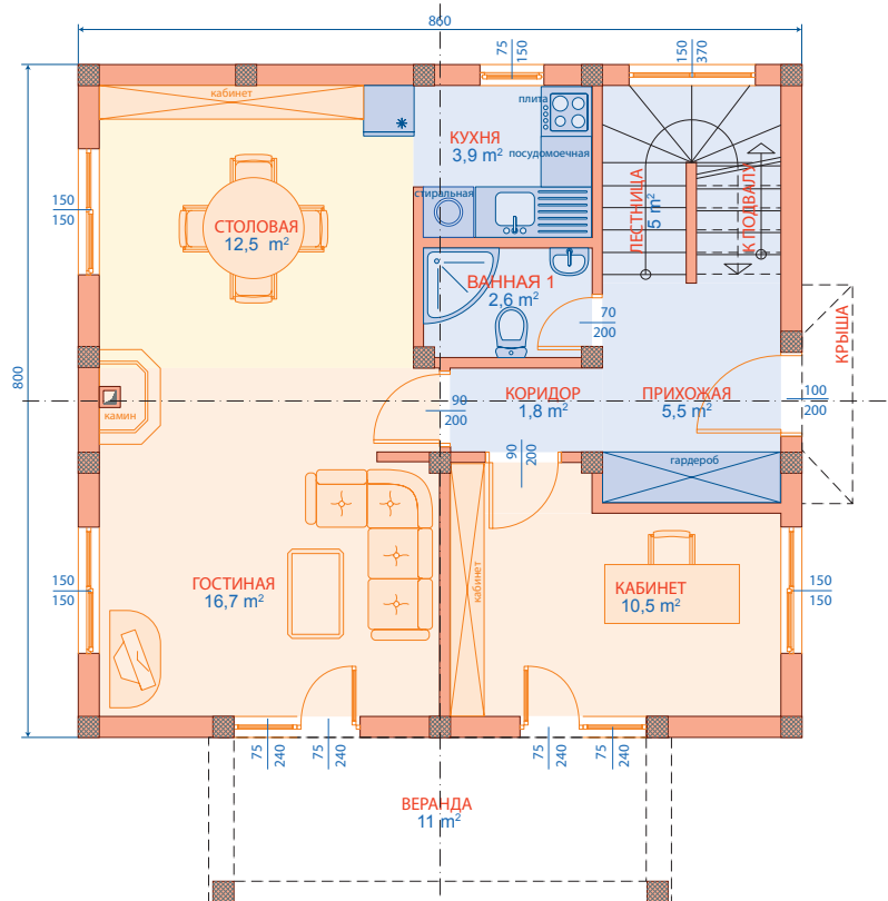
первый этаж площадь: 68,8 м 2 веранда - 11.0 кв.м РПЗ: 174 м 2
