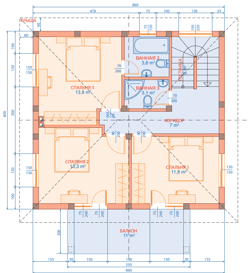
второй этаж площадь: 79,8 м 2 РПЗ: 174 м 2
